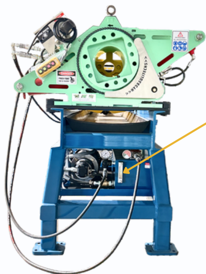
SPU, Unité de puissance standard pour HTW50 glisse sous la table
